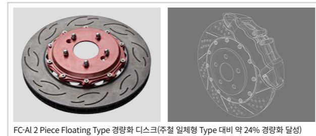
FC-Al 2 Piece Floating Type 경량화 디스크(주철 일체형 Type 대비 약 24% 경량화 달성)
